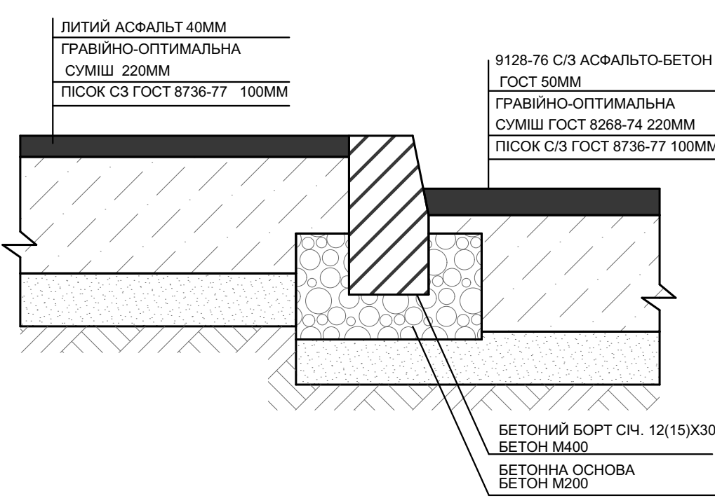
Вузол А М1:5
