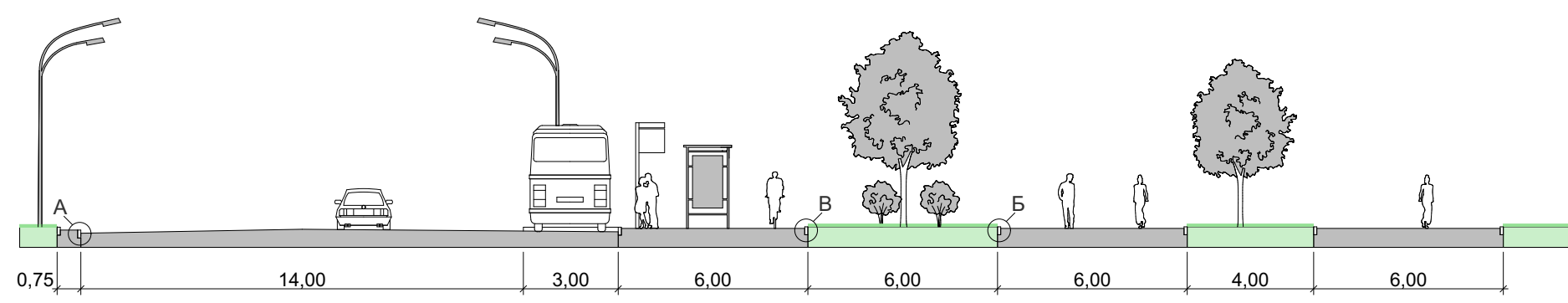
Фрагмент поперозного профілю вулиці Б-Б М1:20
