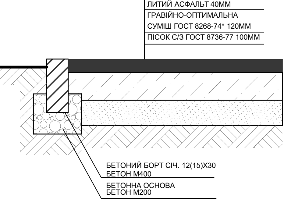
Вузол Б М1:2
