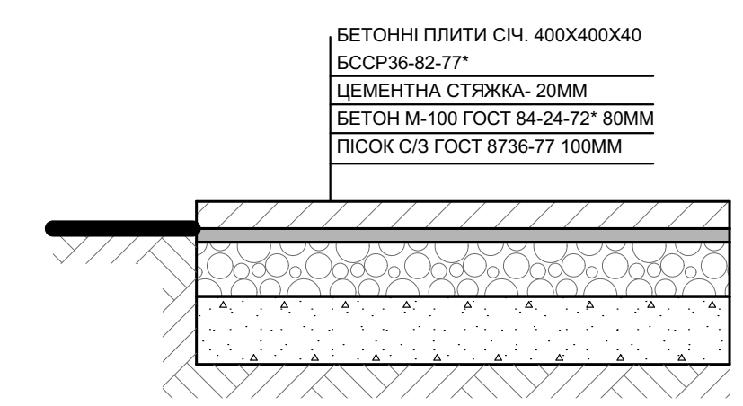
Вузол Б М1:2
