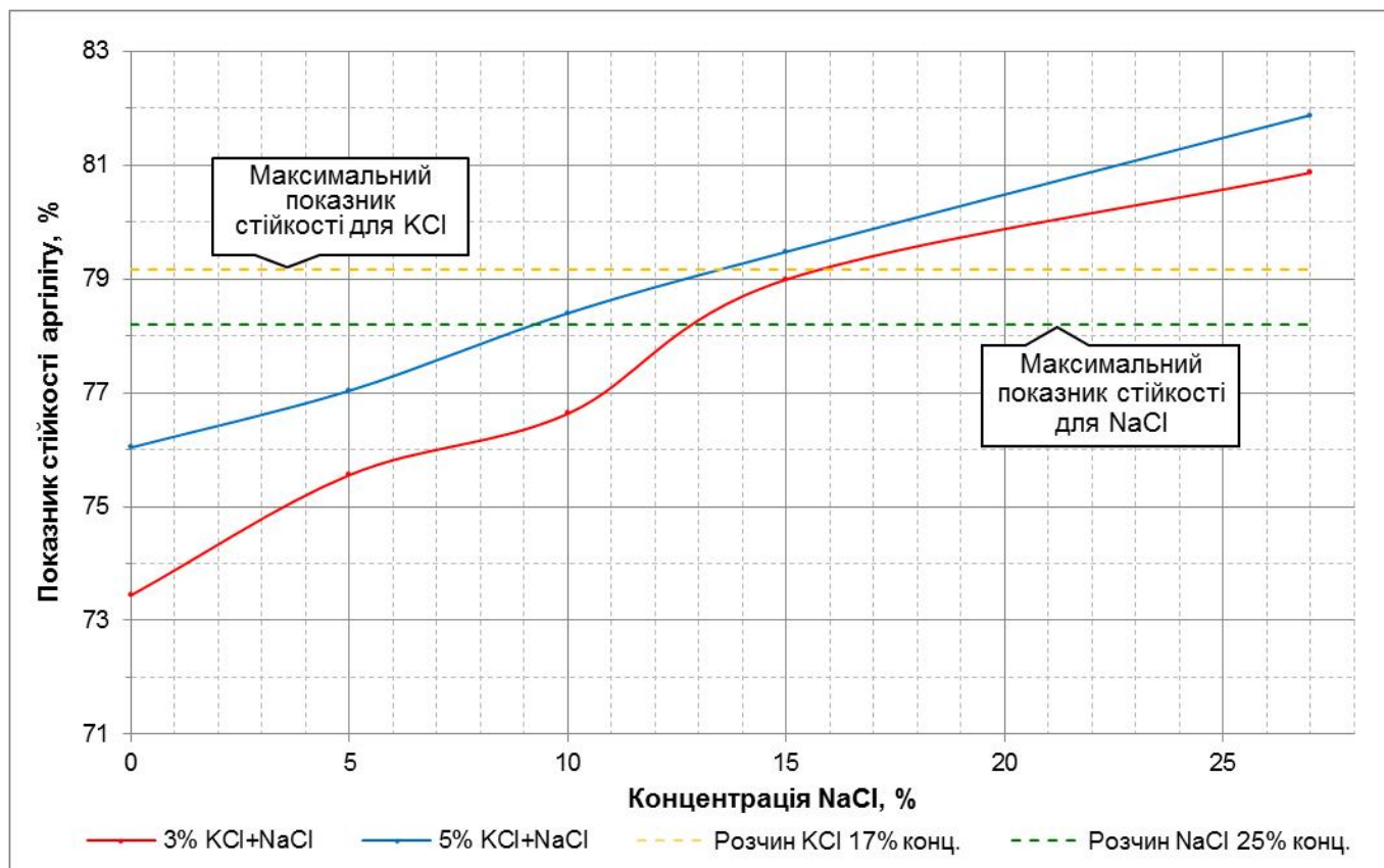
Рисунок 3 – Підвищення стійкості аргіліту (Rolling Test) при спільному застосуванні хлоридів калію і натрію
