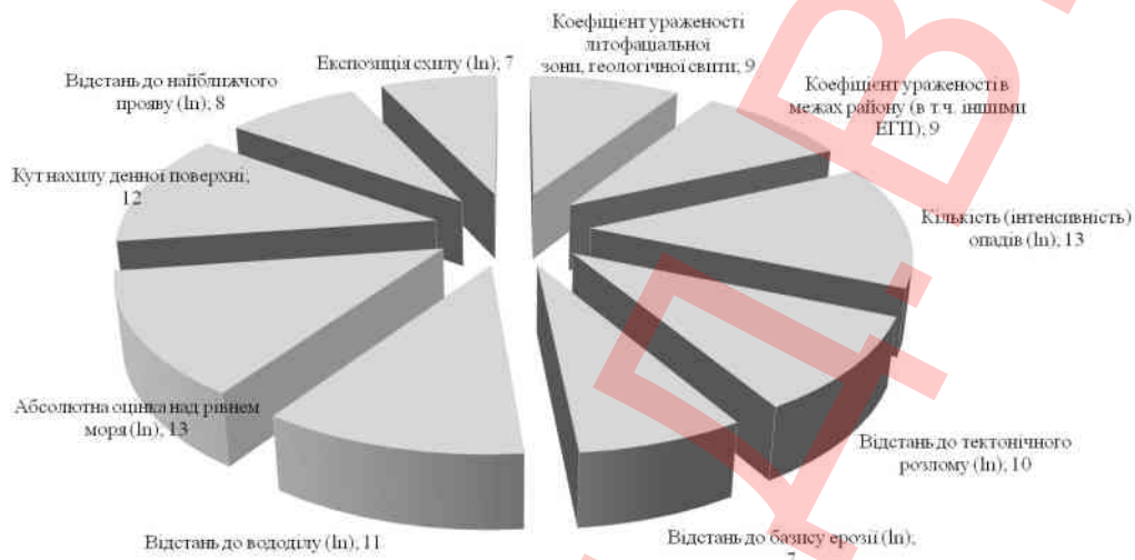
Рис. 4.3. Вагові коефіцієнт інформативності факторних характеристик для природної складової, %
