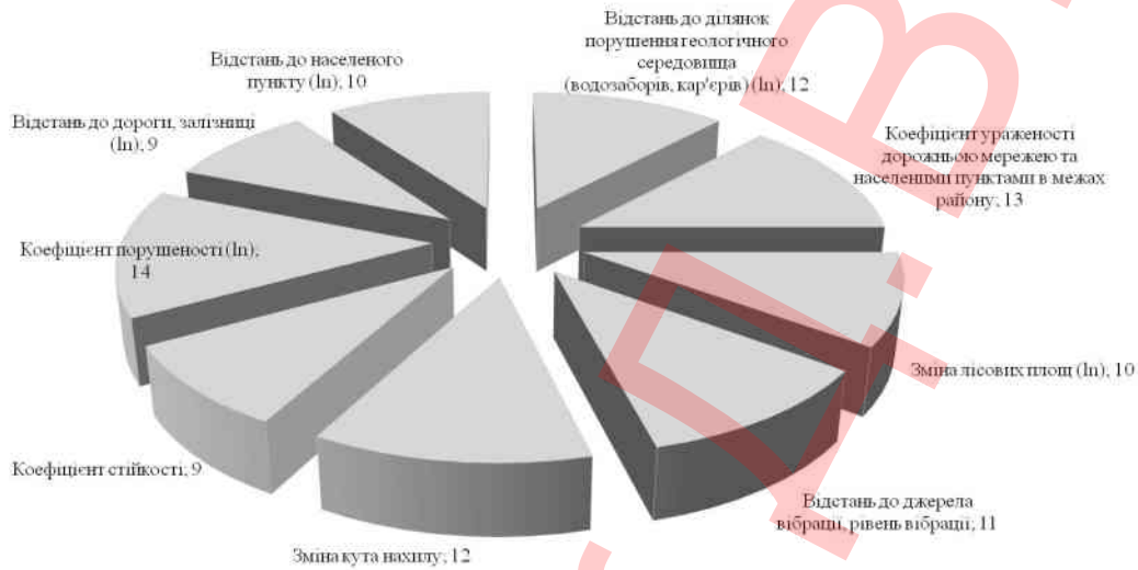
Рис. 4.5. Вагові коефіцієнт інформативності факторних характеристик для техногенної складової, %
