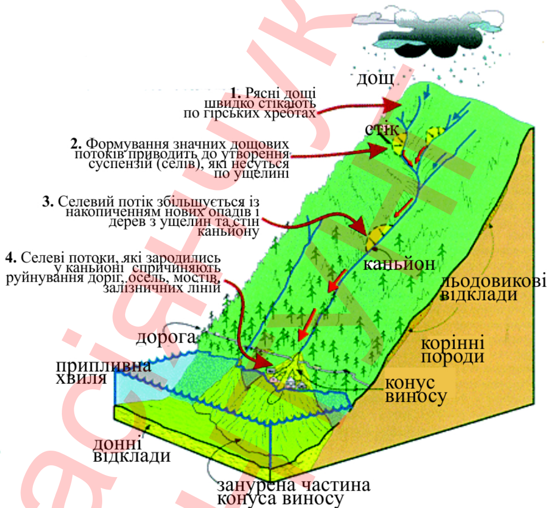
Рис. 2.4. Селевий потік (модель за Джозефом Оконелом та Джеймі Фліпплейсоном)
