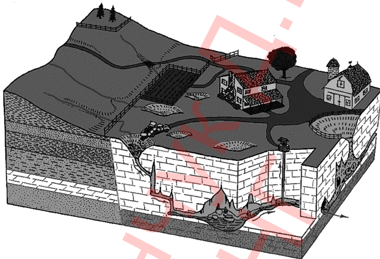
Рис. 2.5. – Карстові процеси (модель за Максимовичом М.К.)
