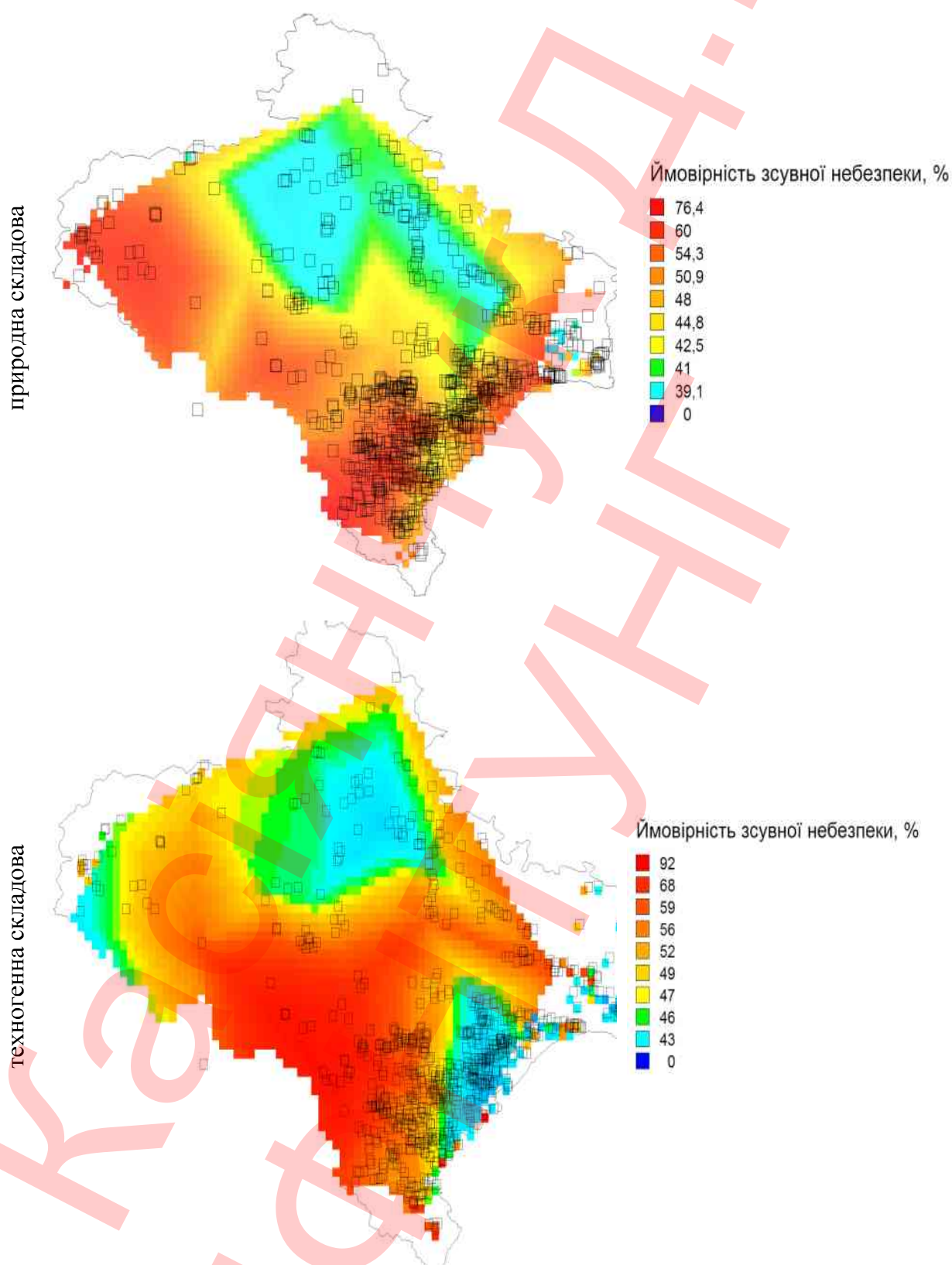
Рис. 5.5. Схематична карта ймовірності зсувної небезпеки для території Івано-Франківської області (для різних складових)
