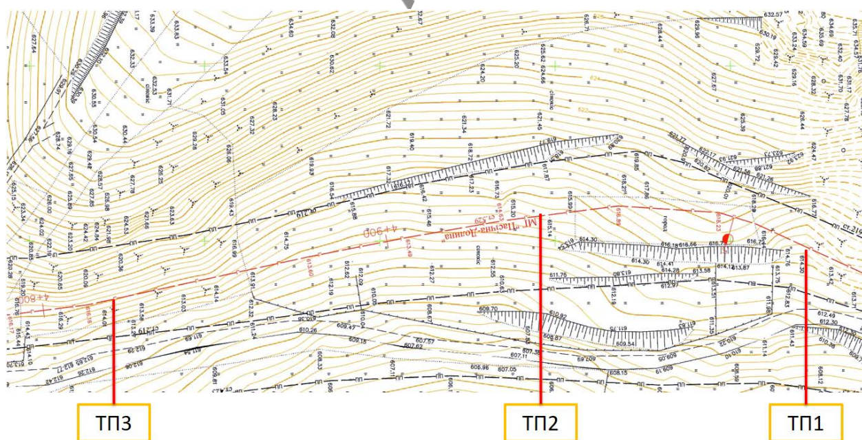
Рисунок 4 - Фрагмент топографічної карти геодезичної зйомки положення магістрального газопроводу «Пасічна-Долина» Ду 500 на 5,1 км
