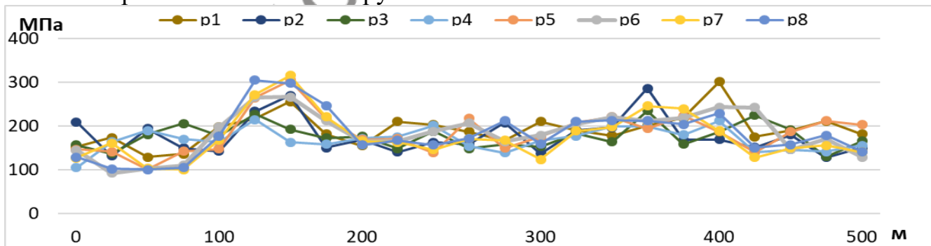
а) Фактичні значення напружень
