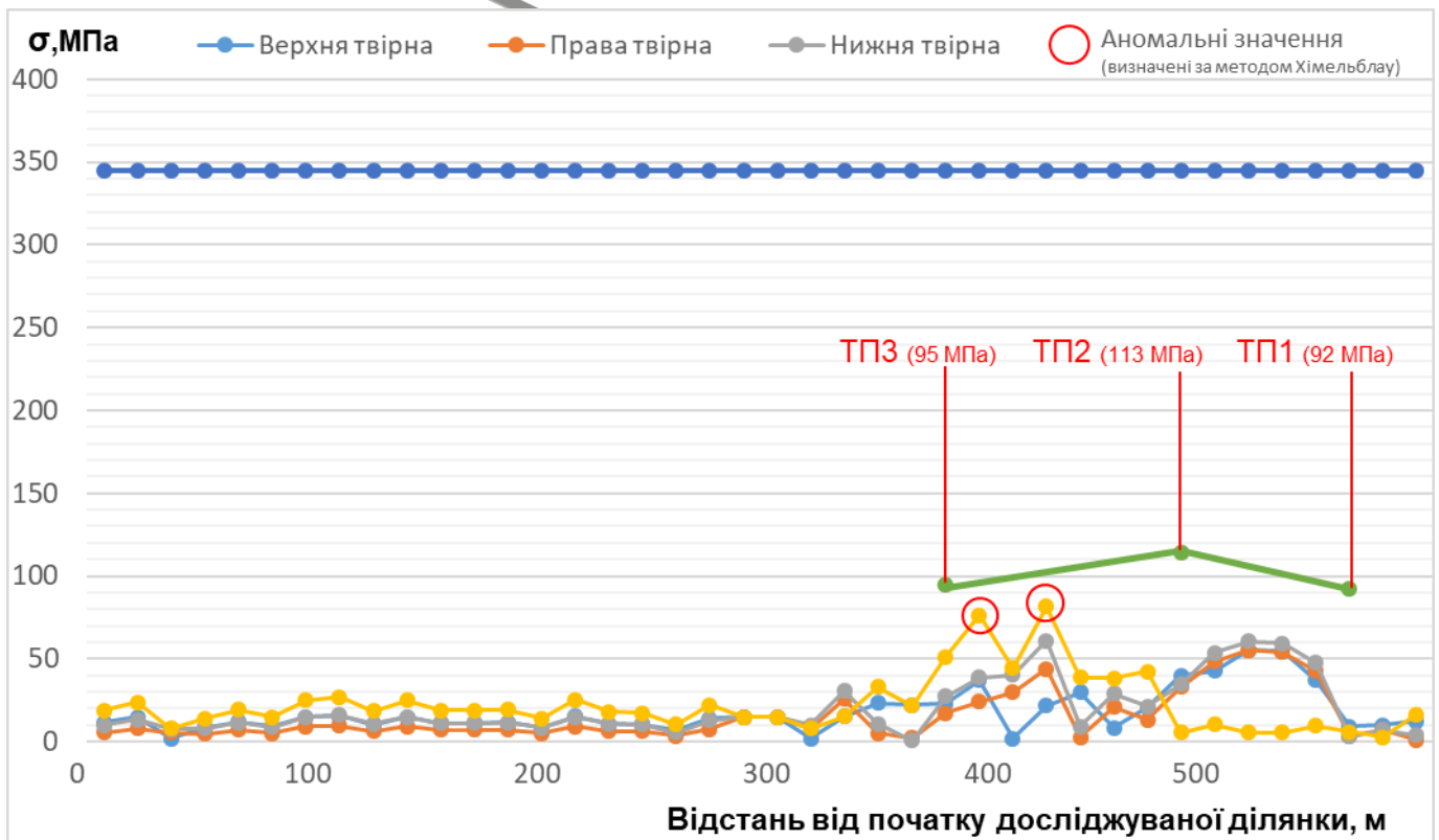
Рис. 6 Графік зміни напружень труби досліджуваної ділянки газопроводу «Пасічна-Долина» Ду500 протяжністю 800 м
