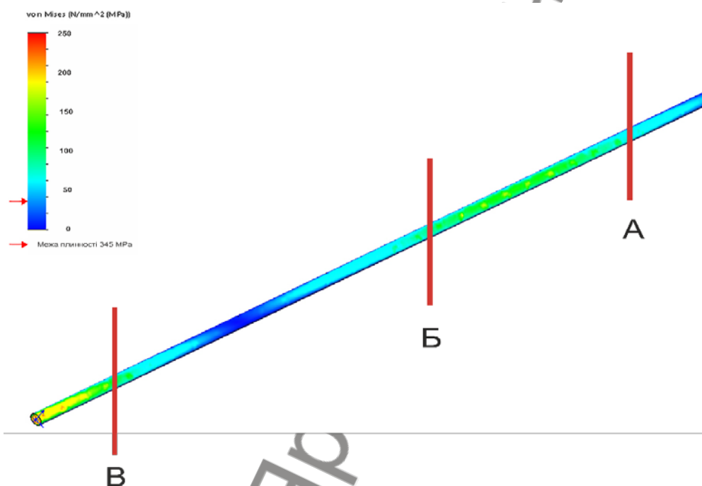
Рисунок 8 - Моделювання розрахованого НДС ділянки газопроводу «Пасічна-Долина» Ду 500 у середовищі SolidWorks
