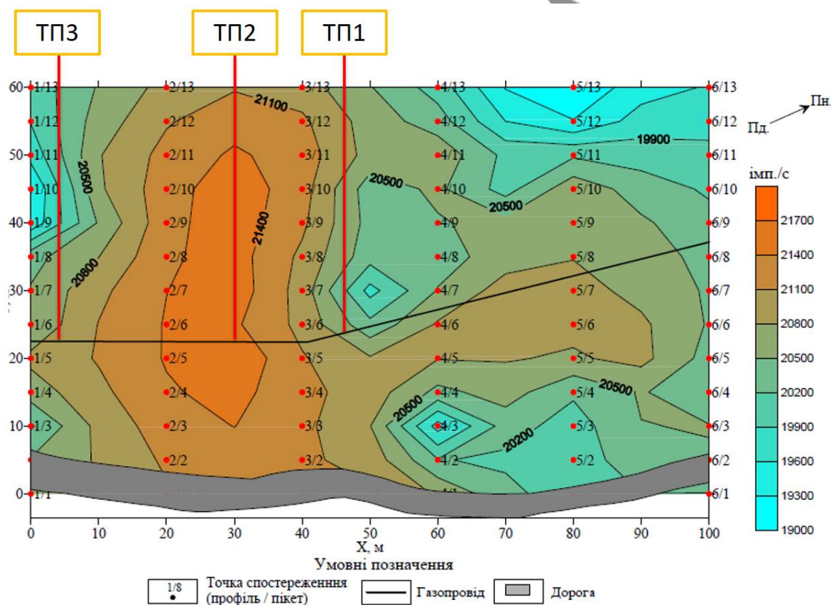
Рисунок 9 - Карта інтенсивності природного імпульсного електромагнітного поля Землі (горизонтальна складова, напрям антени впоперек схилу). Масштаб 1:500
