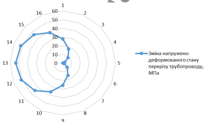
Рисунок 7 - Розподіл напружень в поперечному сеченні труби газопроводу «Пасічна-Долина» Ду 500 на відмітці 500 м
