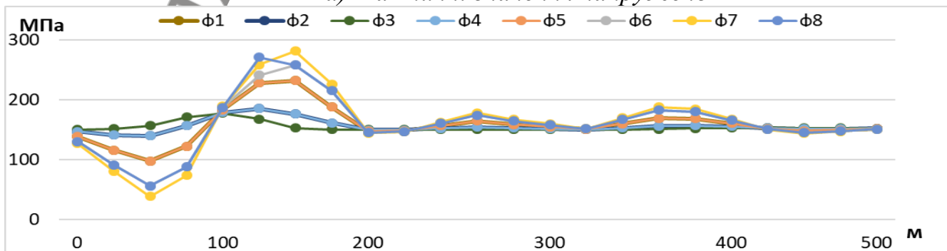
б) Розраховані значення напружень
